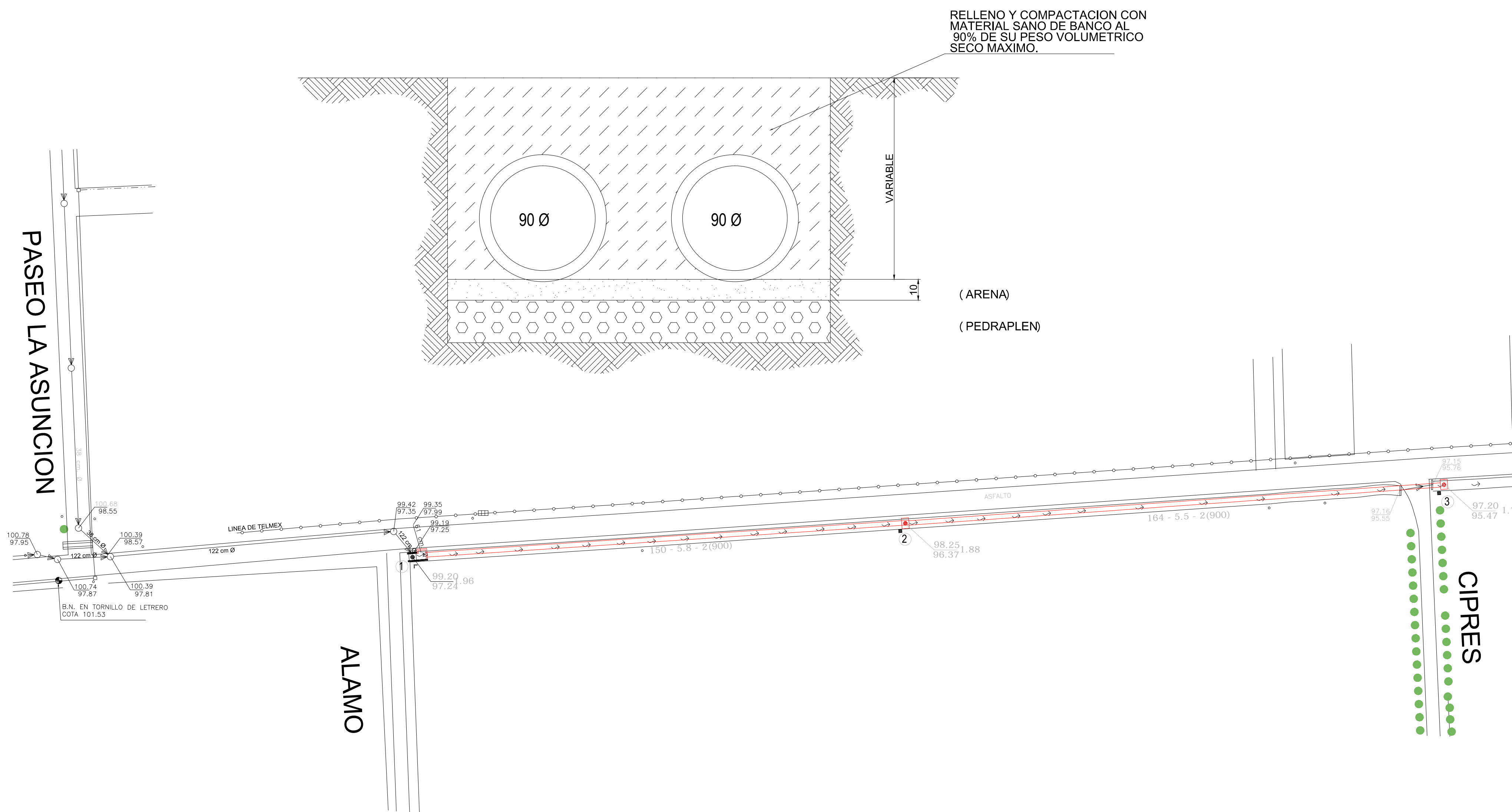
PLANTA COLECTOR PLUVIAL.
